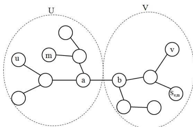
شکل ۱. افراز مجموعه راس‌های درخت T به فرم \Lambda(u, v) = (U, V) متناظر با دو راس u, v . e = (a, b) بال مرکزی مربوط به u, v فرض شده است
